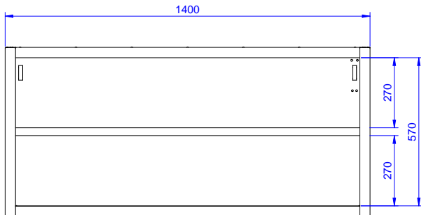
Front aanzicht
